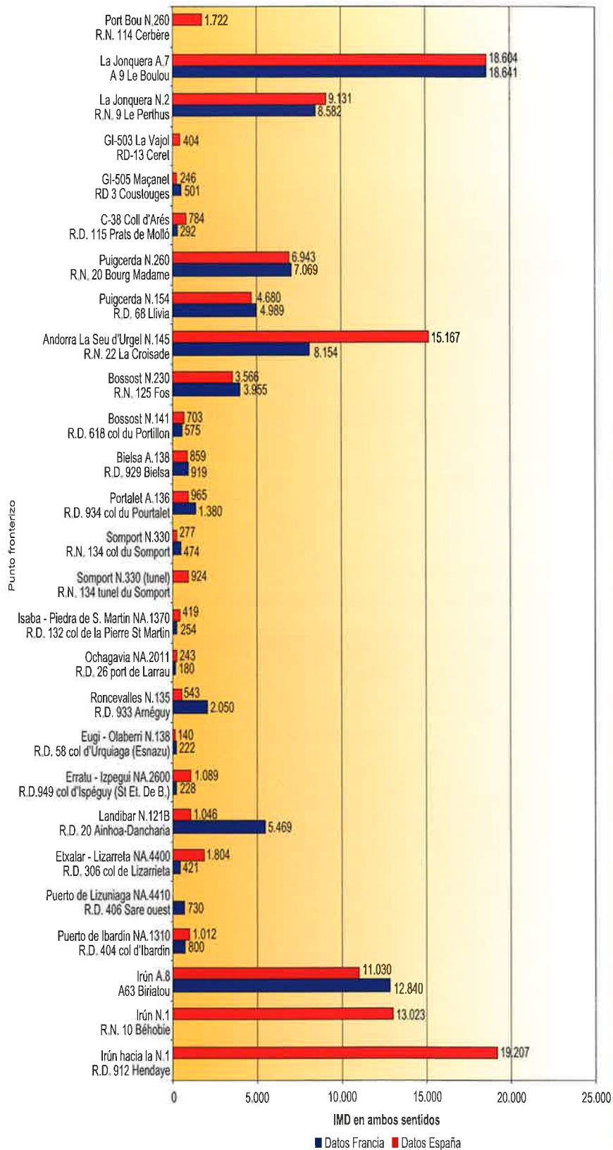
IMD de vehículos ligeros (en ambos sentidos). Año 2003
