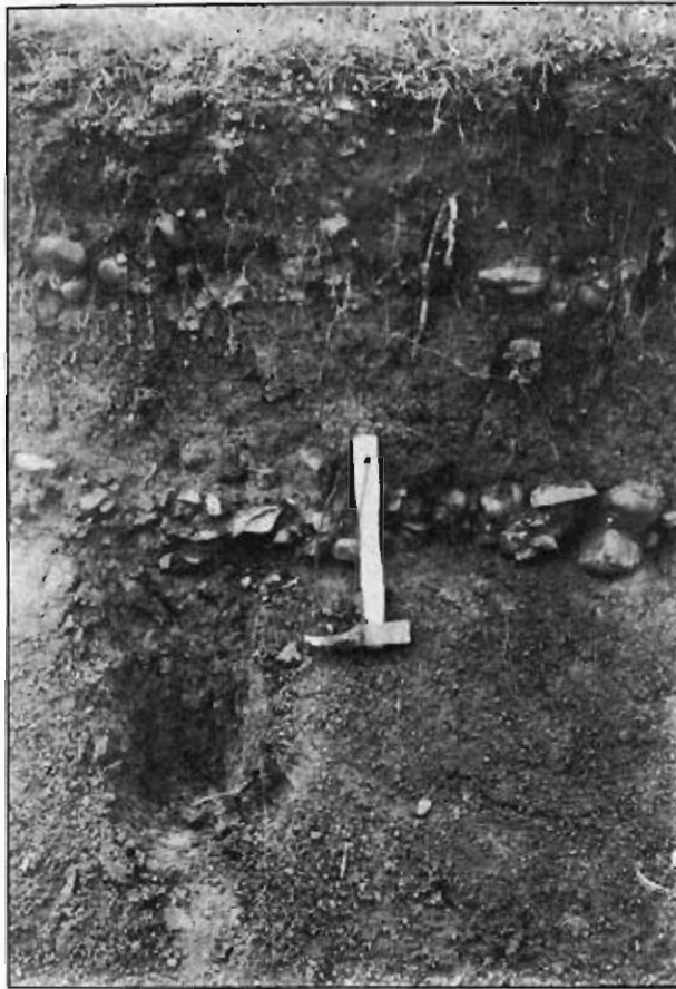
Fig. 3.7.— Detalle del grupo A2 en el arroyo de la Solanilla. (Hoja 162-4).
