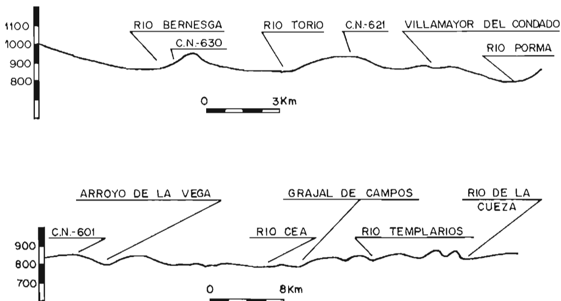
Fig. 2.1.— Perfiles topográficos representativos del Tramo.
