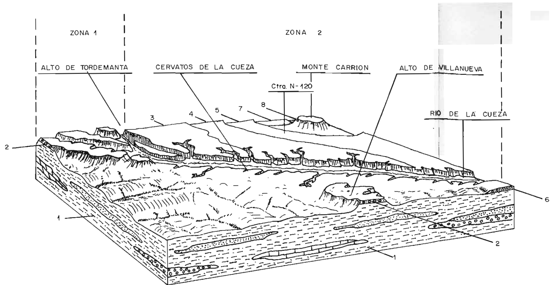
BLOQUE - DIAGRAMA ESQUEMATICO PARCIAL DE LAS ZONAS 1 y 2 1: 321a ; 2: 350 ; 3: T6 ; 4: T5 ; 5: T4 ; 6: T3 ; 7: T2 ; 8: T1
