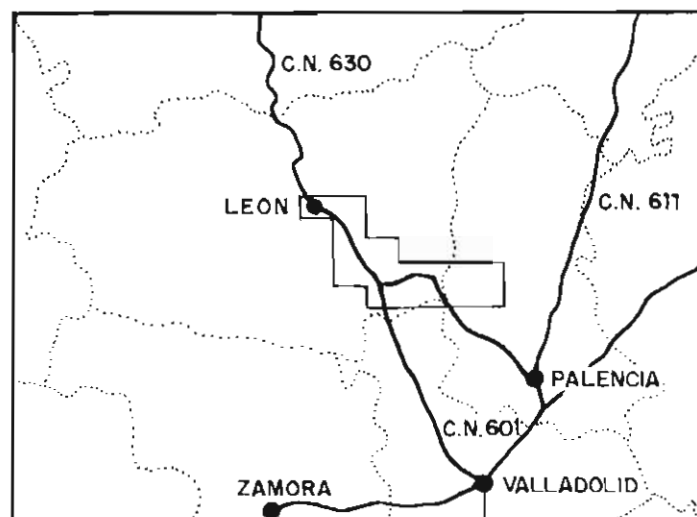
Fig. 1.1.— Esquema de situación del Tramo.
