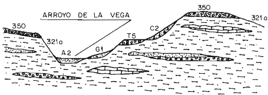
Fig. 3.31. — Corte geológico esquemático del grupo G1 en el arroyo de la Vega (Hoja 233-1).
