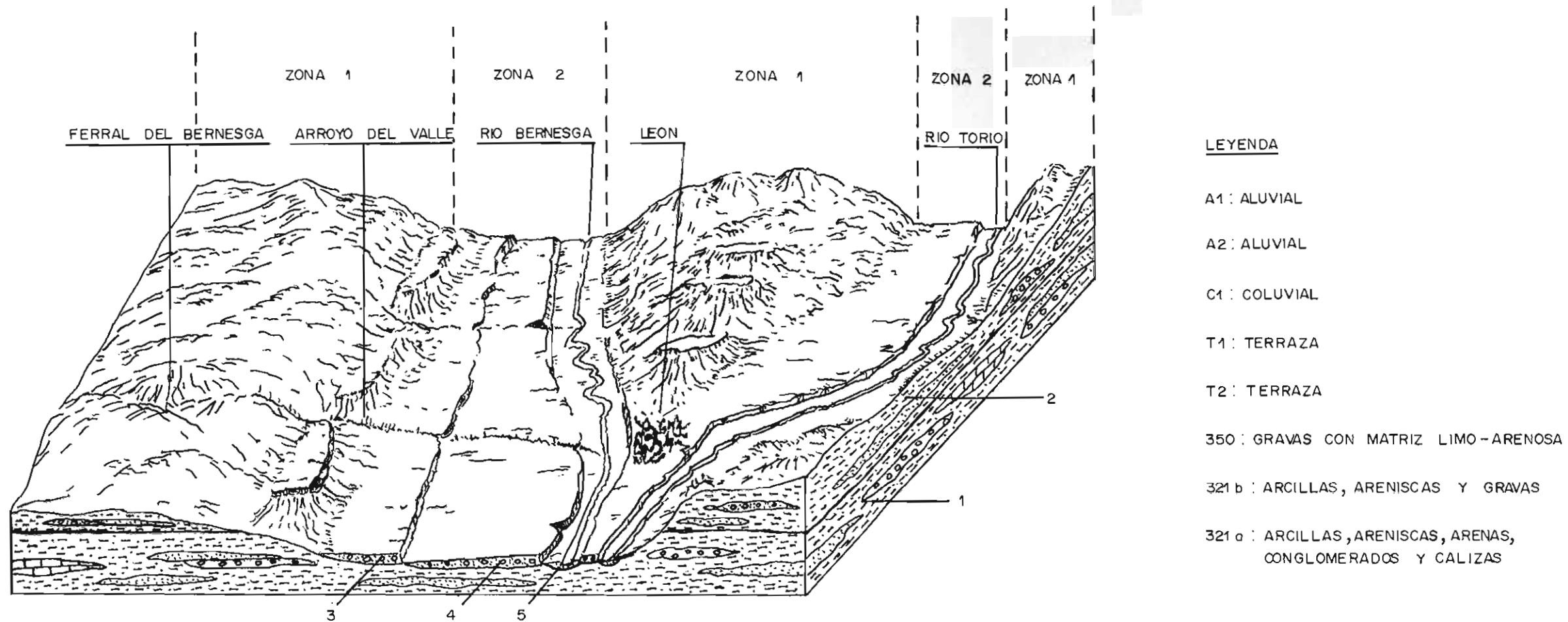
BLOQUE-DIAGRAMA ESQUEMATICO PARCIAL DE LAS ZONAS 1 y 2 1: 321 a; 2: 321 b; 3: T2; 4: T1; 5: A1
