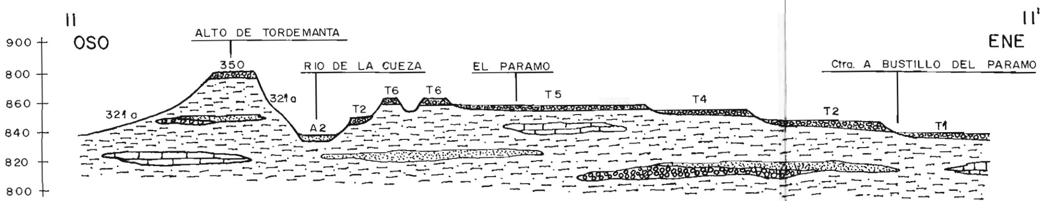
CORTES GEOLOGICOS ESQUEMATICOS DE LA ZONA 2
