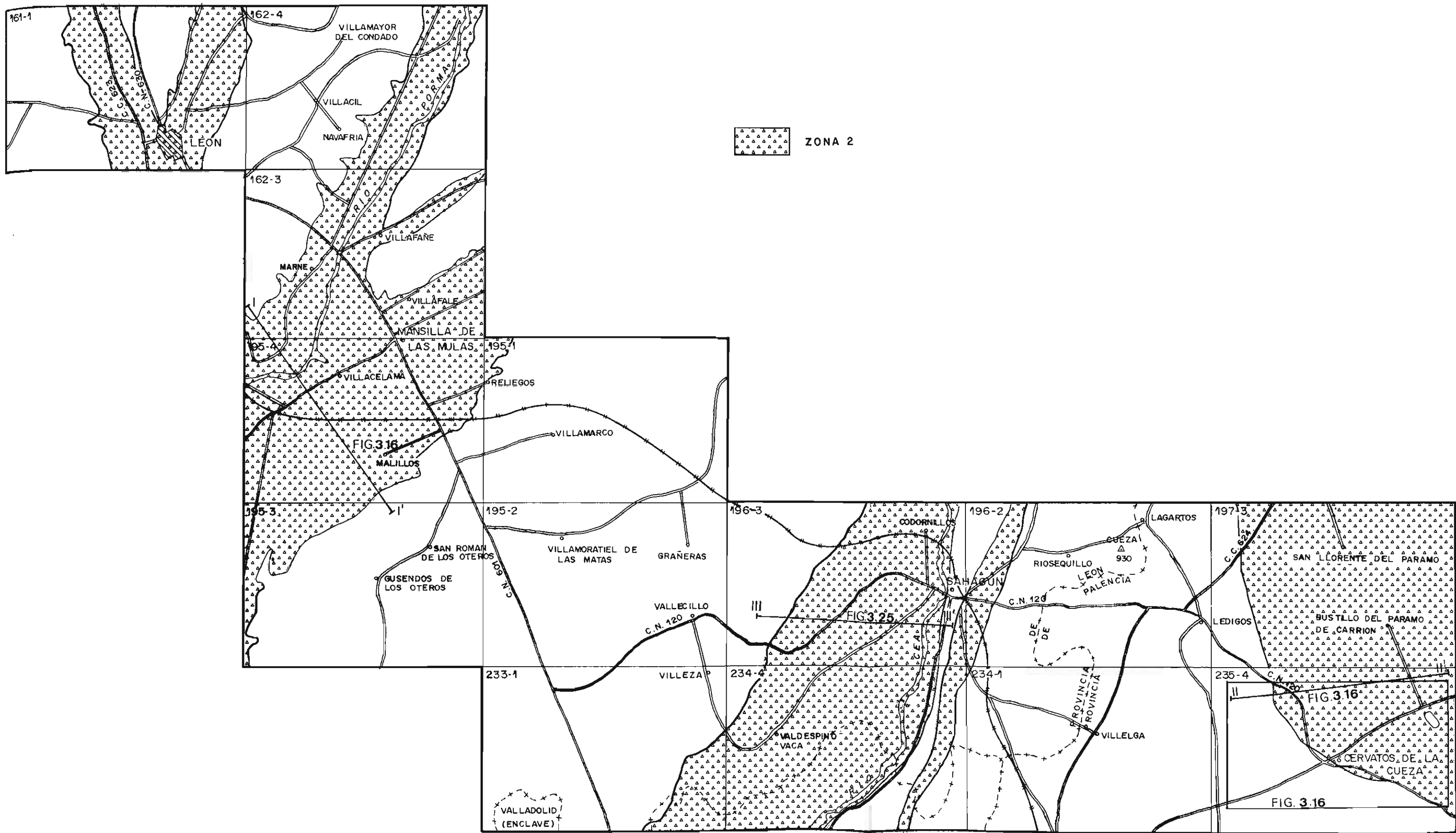
Fig. 3.15.— Esquema de situación de la Zona 2, de un bloque-diagrama y de tres cortes geológicos realizados en la misma.
