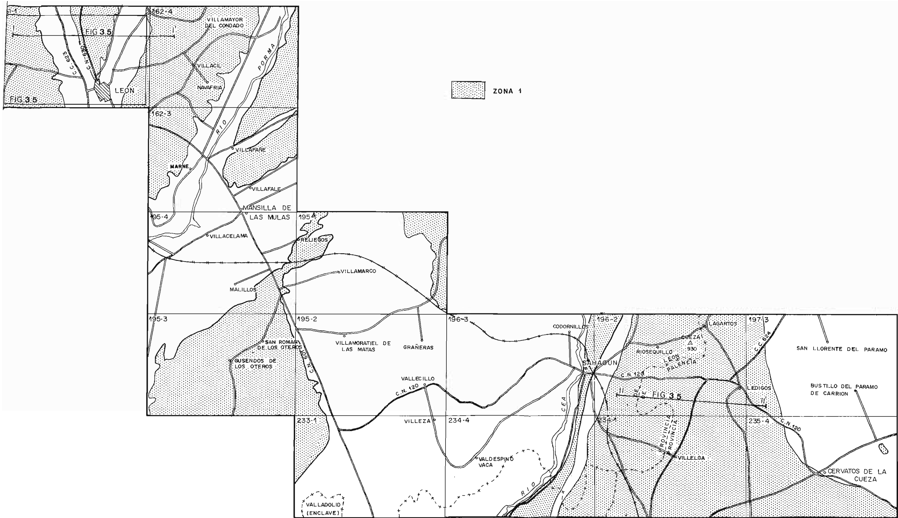
Fig. 3.3.— Esquema de situación de la Zona 1, de un bloque-diagrama y de dos cortes geológicos esquemáticos realizados en la misma.
