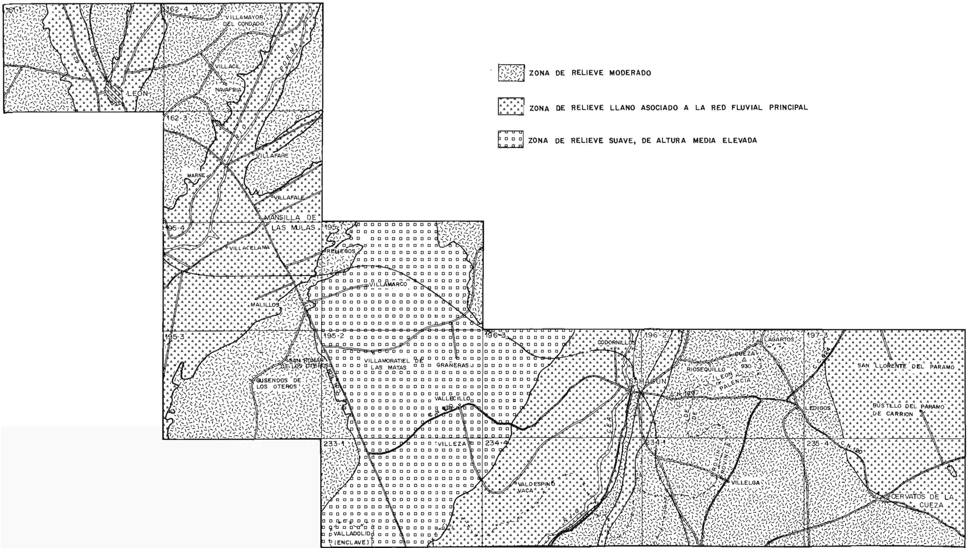
Fig. 2.2.— División del Tramo en zonas desde el punto de vista de la geomorfología.
