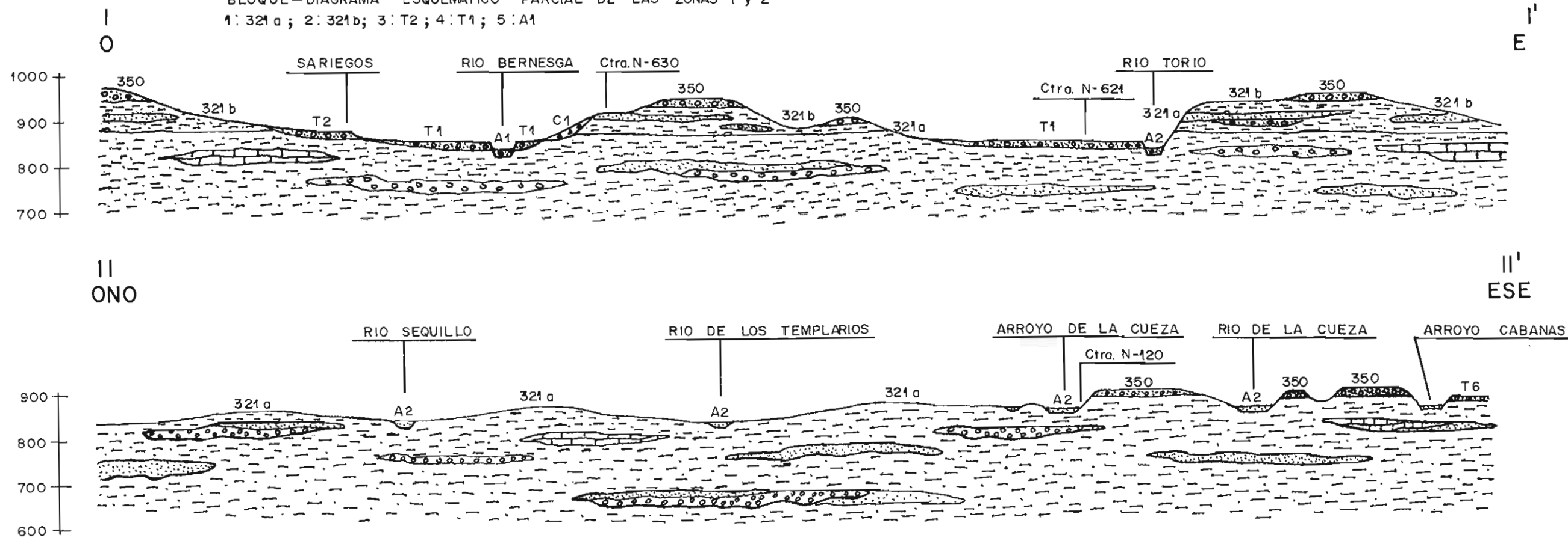
CORTES GEOLOGICOS ESQUEMATICOS DE LA ZONA 1
