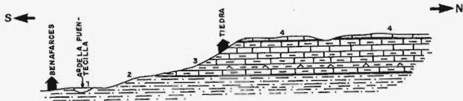
Fig. 6. Esquema geomorfológico de las cuestas miocenas de Pedrosa del Rey-Vezdemarbán.
