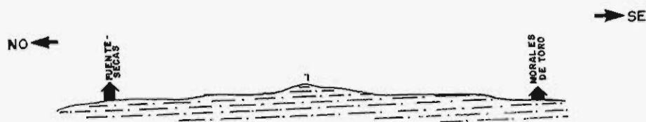
Fig. 5. Esquema geomorfológico de la divisoria miocena de Morales de Toro-Bustillo del Oro.
