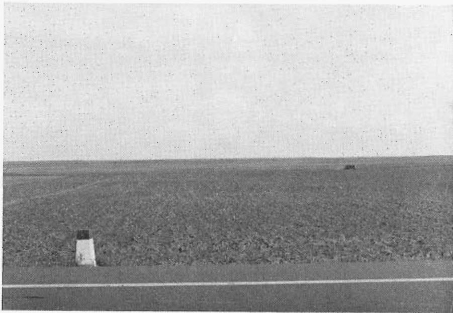
Fot. 3. Vista hacia el Oeste desde la carretera N-VI, Madrid-La Coruña, de los replanos de S. Esteban del Molar.
