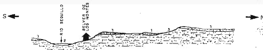
Fig. 4. Esquema geomorfológico de los relieves de Belver de los Montes, San Martín de Valderaduey.
