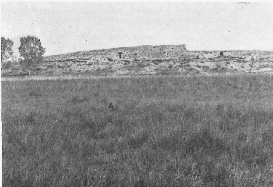
Fot. 16. Niveles de terraza parcialmente cementados (T2) y aluvial arcillo-limoso con arenas dispersas y contenido en materia orgánica (A3), al sur del pueblo de San Román de la Hornija.
