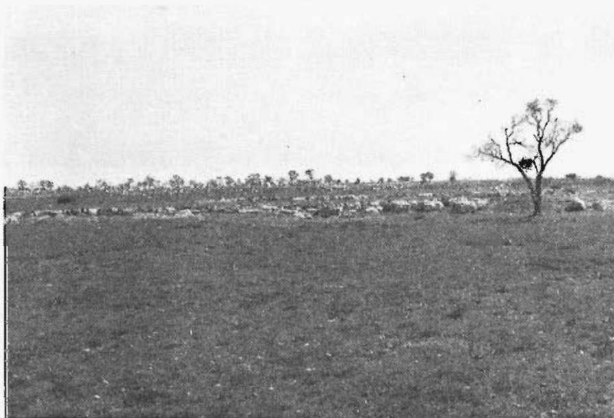
Fot. 37. Afloramientos de la caliza del páramo al norte del pueblo de Tiedra.
