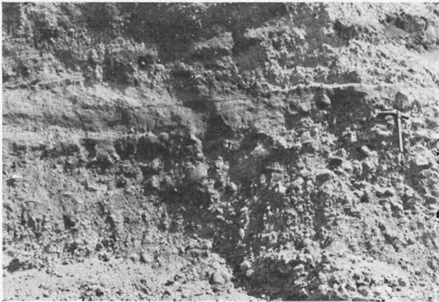
Fot. 43. El nivel de terraza T2, al sur del pueblo de San Román de Hornija
