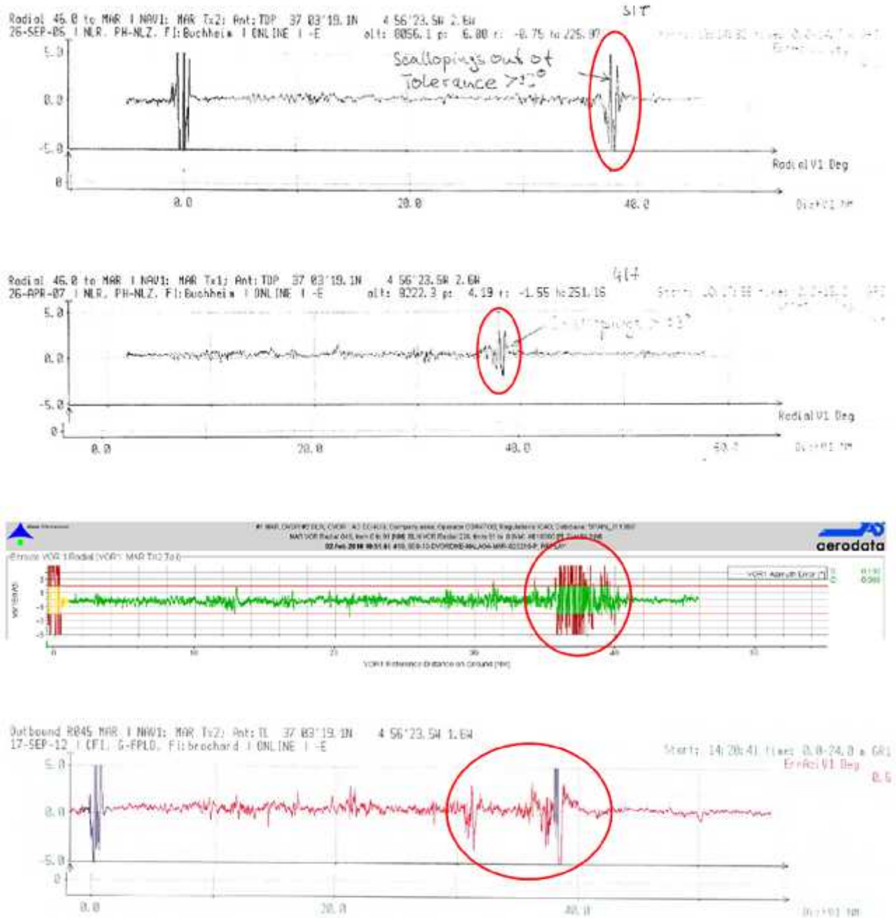
Figura 22. Ejemplo de afecciones a un sistema VOR: registros del radial 046 del DVOR MAR.
