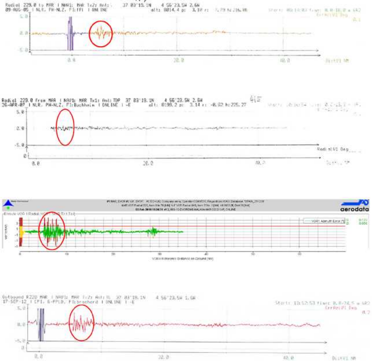
Figura 23. Ejemplo de afecciones a un sistema VOR: registros del radial 229 del DVOR MAR.
