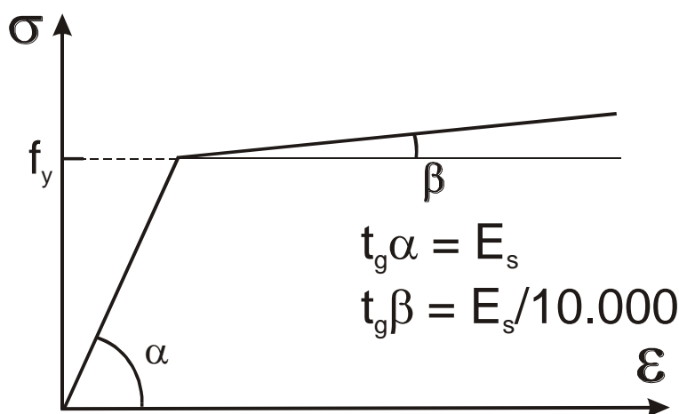
Figura 32.2.b. Diagrama tensión-deformación bilineal, con segunda rama inclinada
